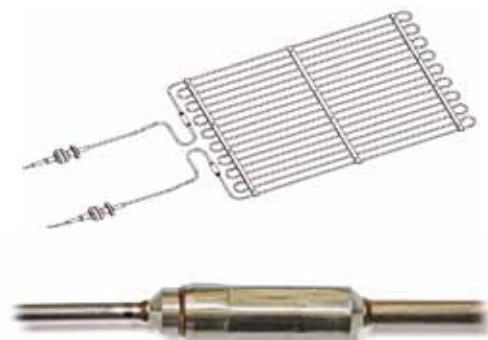
Laser geschweißte Anschluss technik
